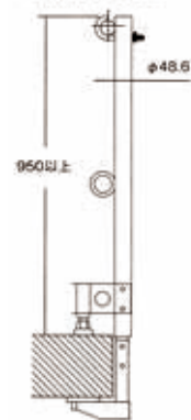
スタンション NRE型
