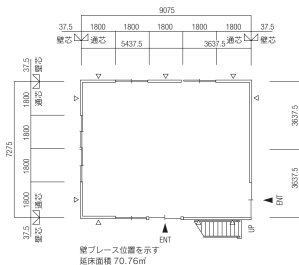
1F 平面図
