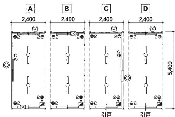
SH-HP54 平面図
