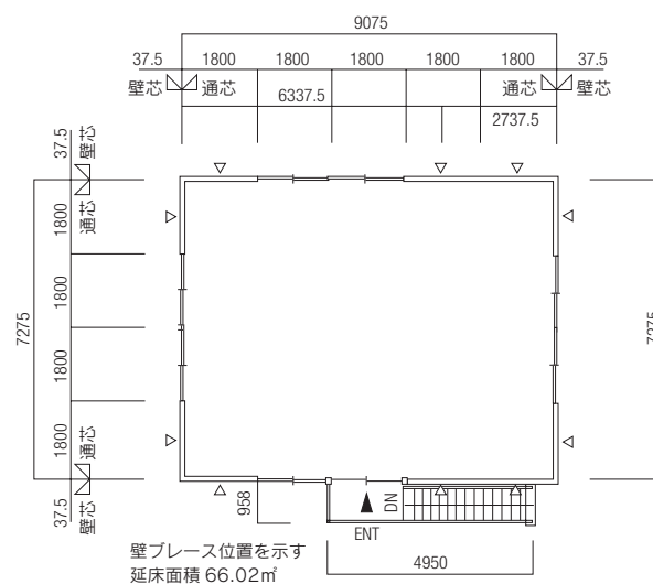
2F 平面図
