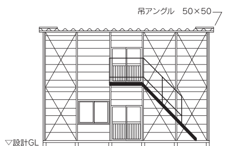
立面図
