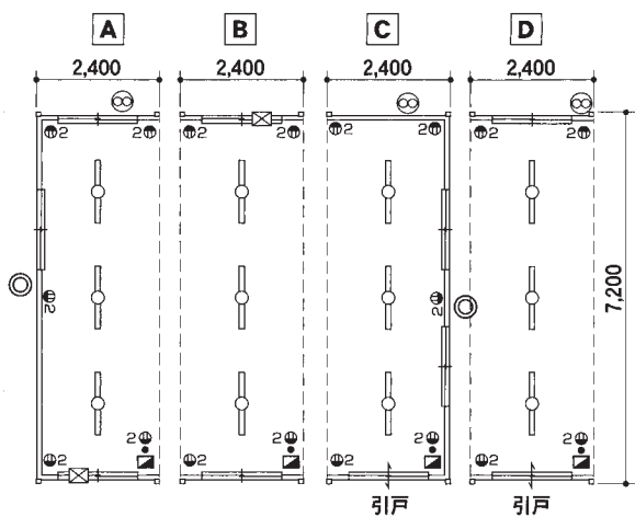
SH-HP72 平面図
