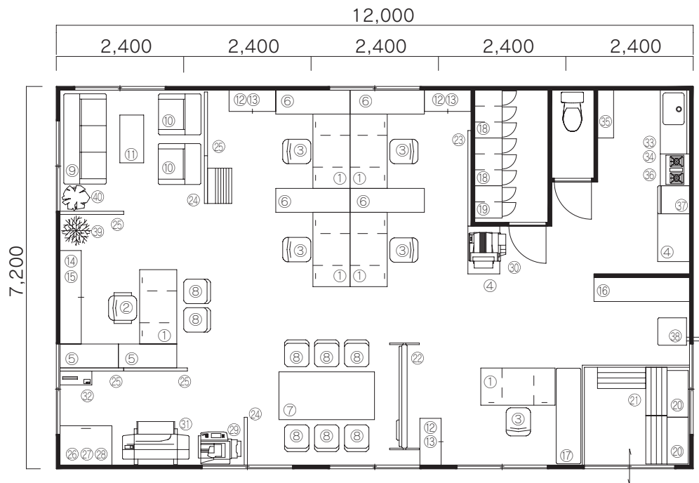
仮設事務所平面図 1/100
