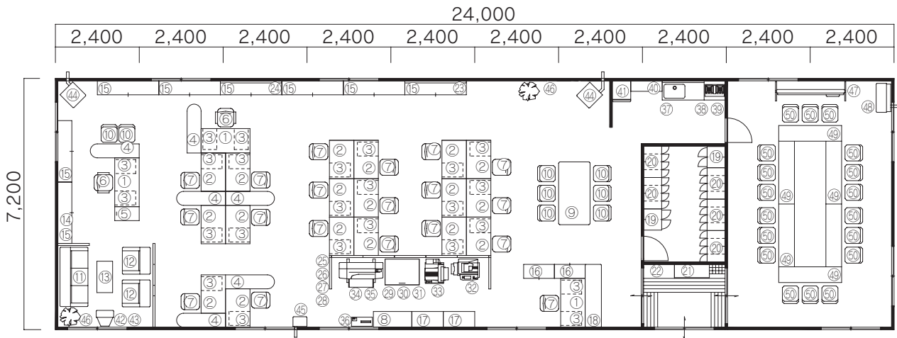
仮設事務所平面図 1/150
