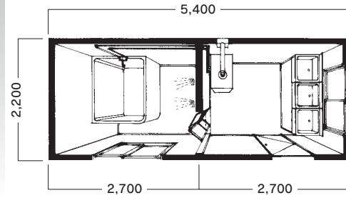
フロハウス B-2型
