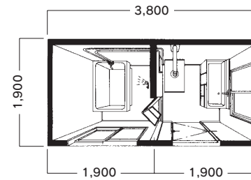
フロハウス B-1型
