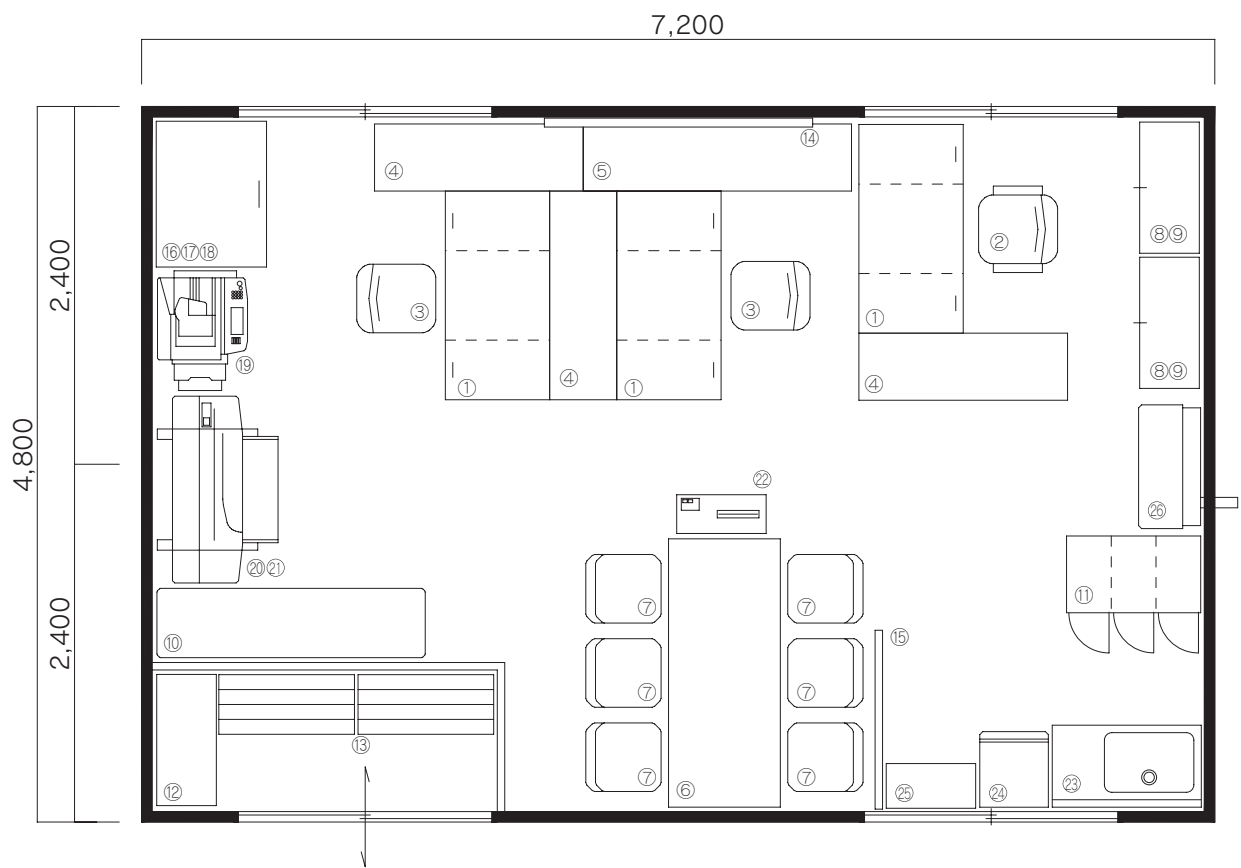
仮設事務所平面図 1/50
